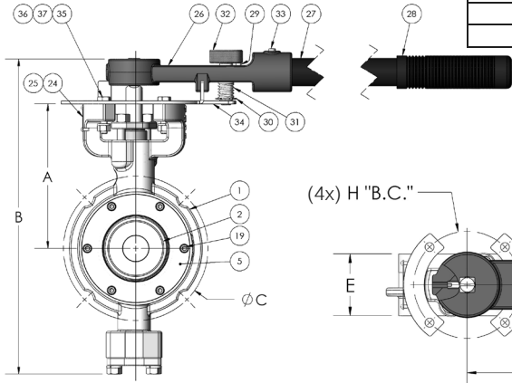
2.5" 150 / 200 WAFER SHOWN
